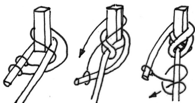
7a. Halvstikk med sikringsstikk er en grei måte å fortøye en liten båt på.
